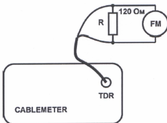
Рисунок 1 - Схема подключения при измерении частоты калибровочных меток.
