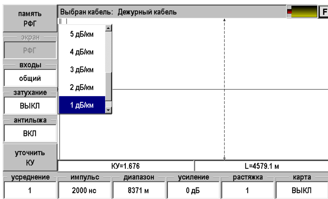
Рис. 14. Функция компенсации затухания.
