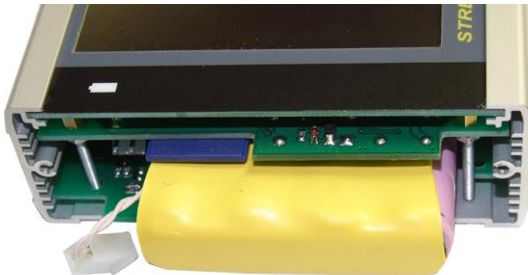
Рис. 4. Аккумуляторный отсек прибора.
