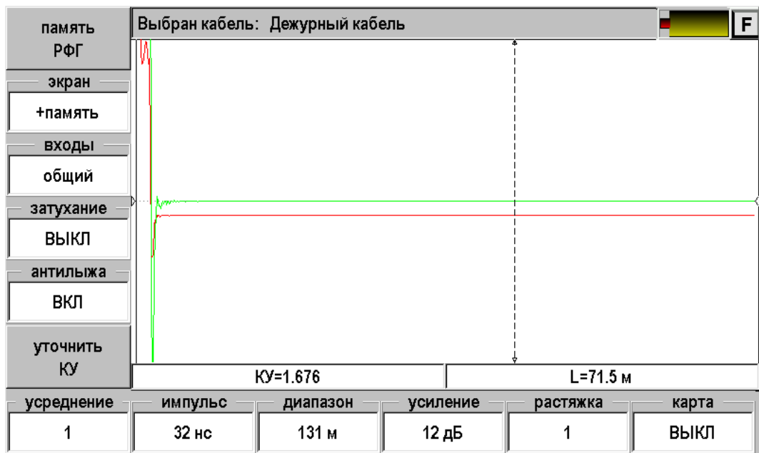
Рис. 18. Сравнение рефлектограмм.
