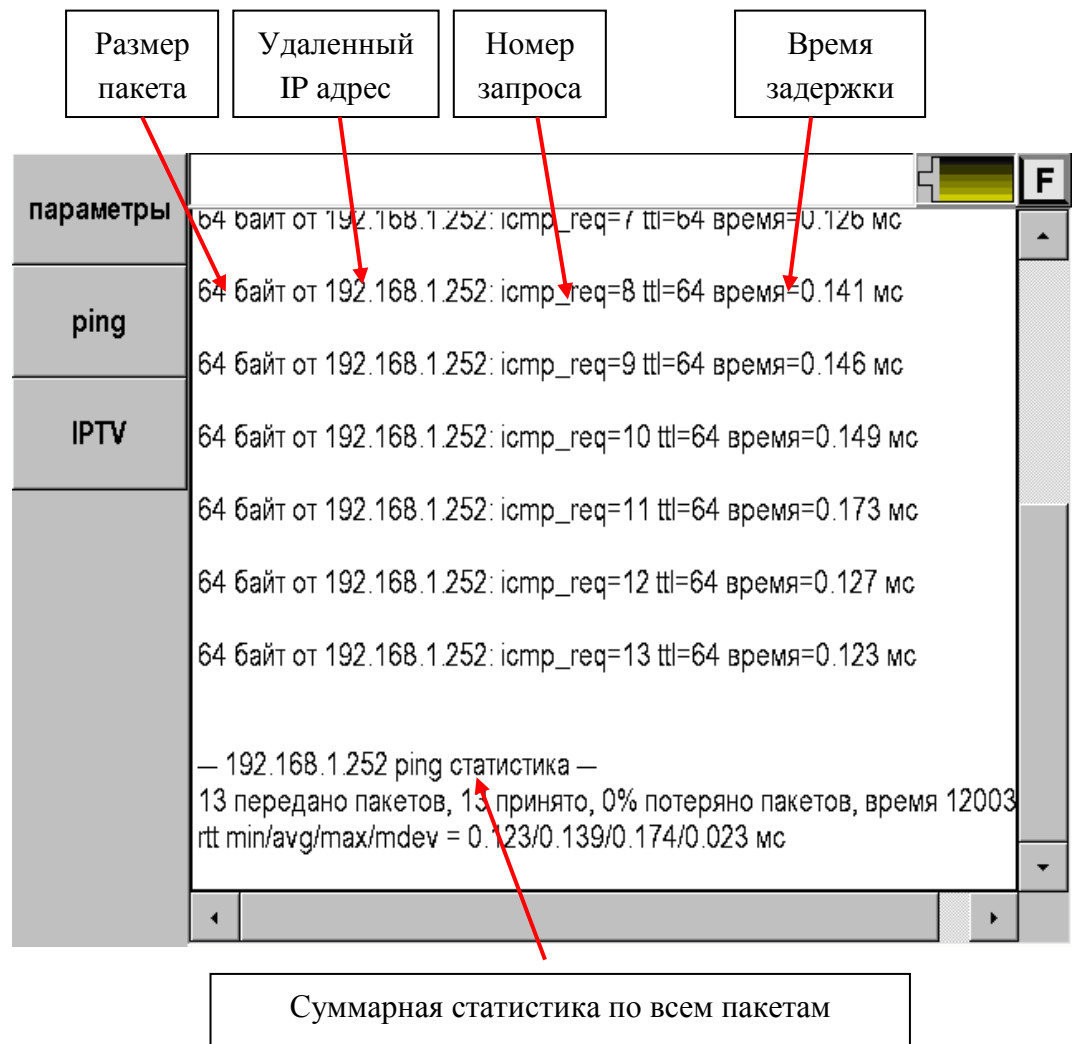
Рис. 39. Результат Ping.
