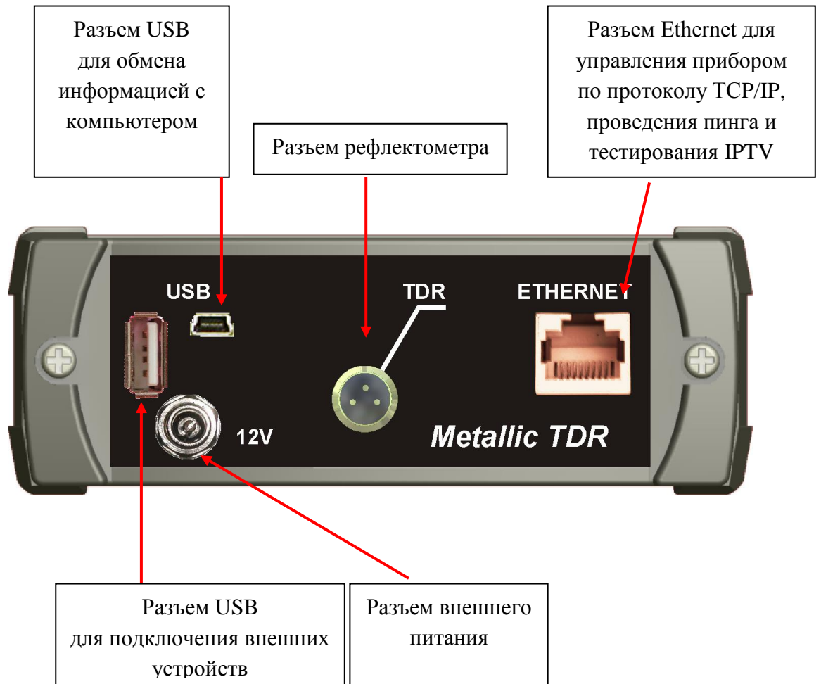
Рис. 2. Внешний вид панели разъемов прибора.
