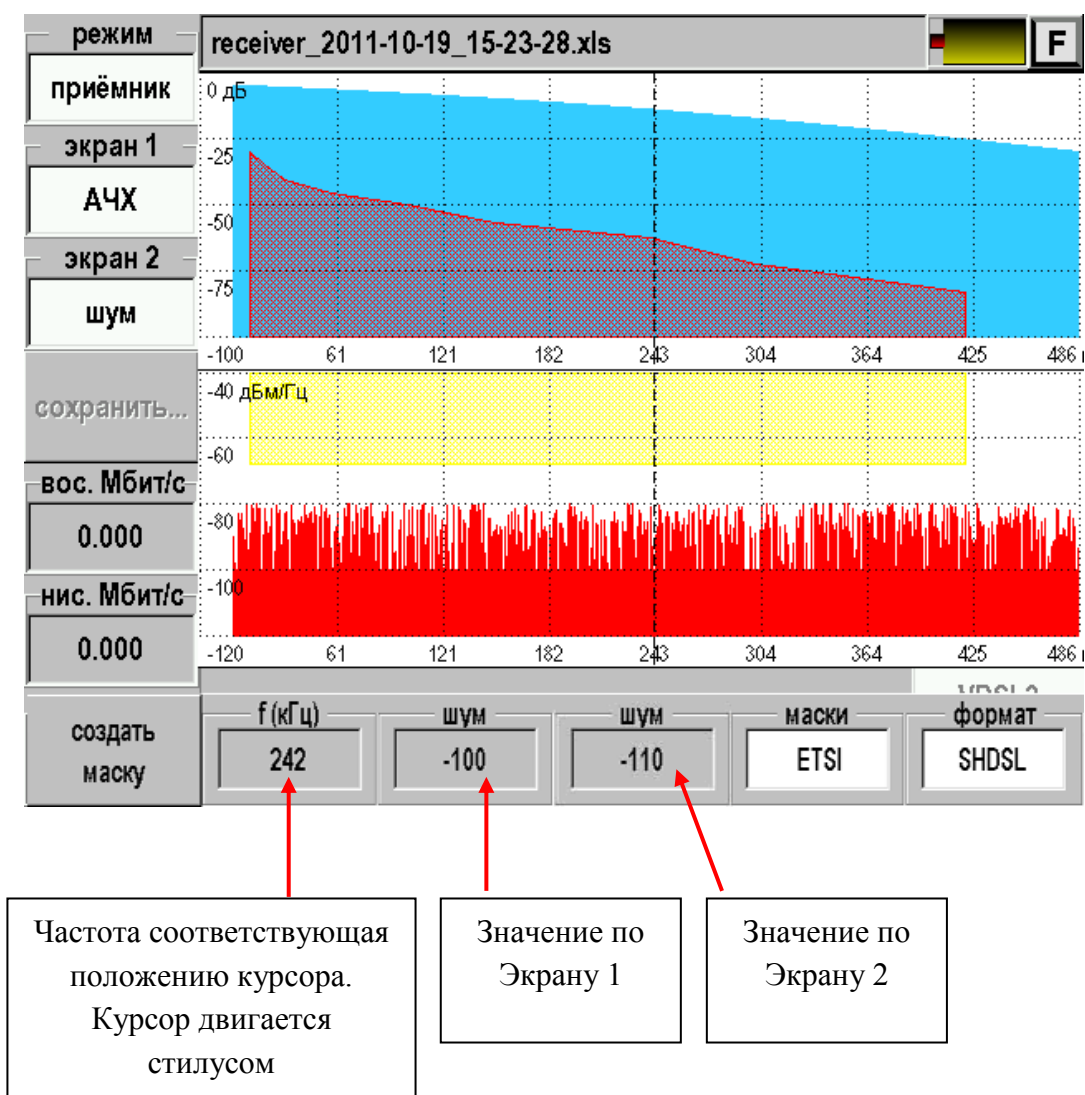
Рис. 24. Приемник. SHDSL.
