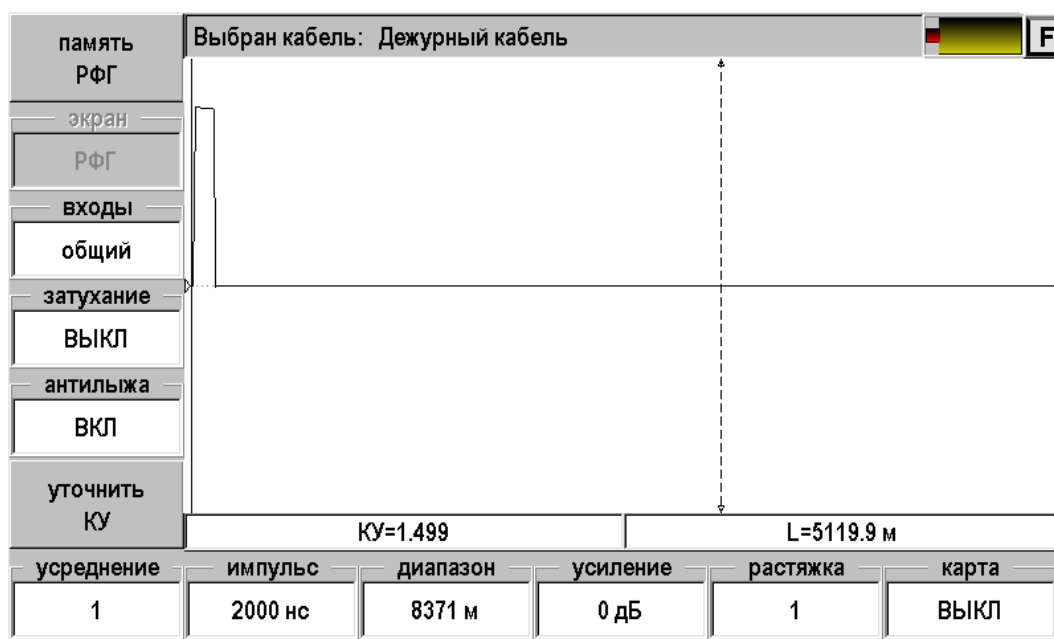
Рис. 9. Экран рефлектометра.
