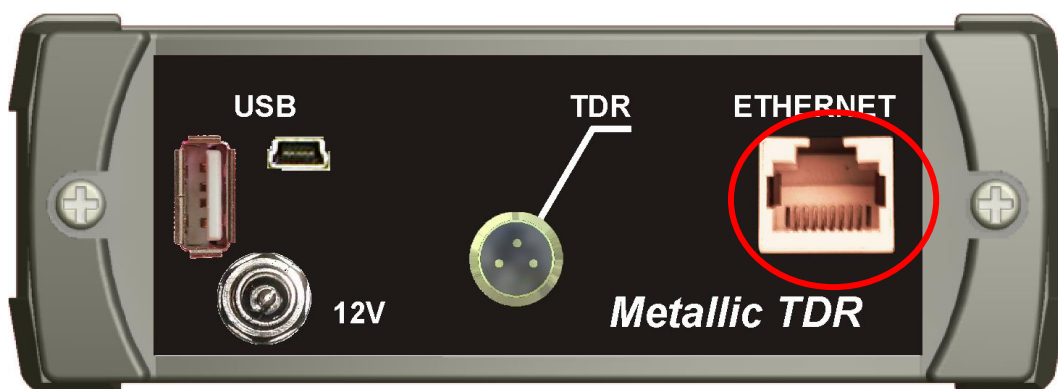
Рис. 36. Разъем Ethernet.
